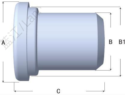
SPR型塞棒
